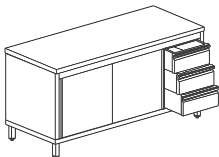
Tavolo armad. scorr. con cassetiera STSCSS600 - STSCSS700
