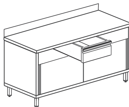
Tavolo armad. scorr. con alzata 1 cassetto STASA/C600 - STASA/C700
