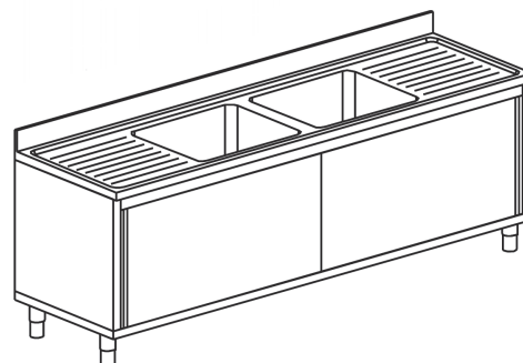
Lavello armadiato scorr. 2 vasche 2 gocc. SLA2V2G600 - SLA2V2G700
