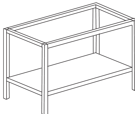
Telaio in tubo 4 gambe con ripiano STTR4G
