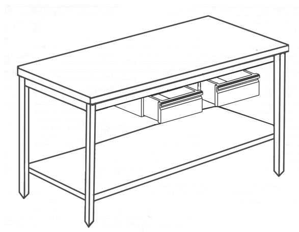
Tavolo a giorno 2 cassetti con ripiano
