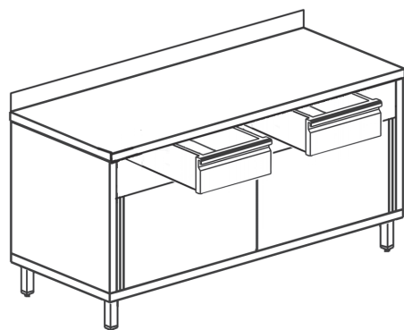
Tavolo armad. scorr. 2 cassetti con alzata STASA/2C600 - STASA/2C700
