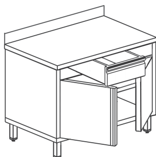
Tavolo armad. 2 batt. con cassetto e alzata STA2BA/C600 - STA2BA/C700
