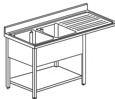
Lavello a sbalzo 2 vasche gocc.
