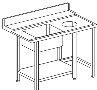
Tavolo entrata lavast. con vasca e foro STEVF
